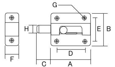
寸法図
